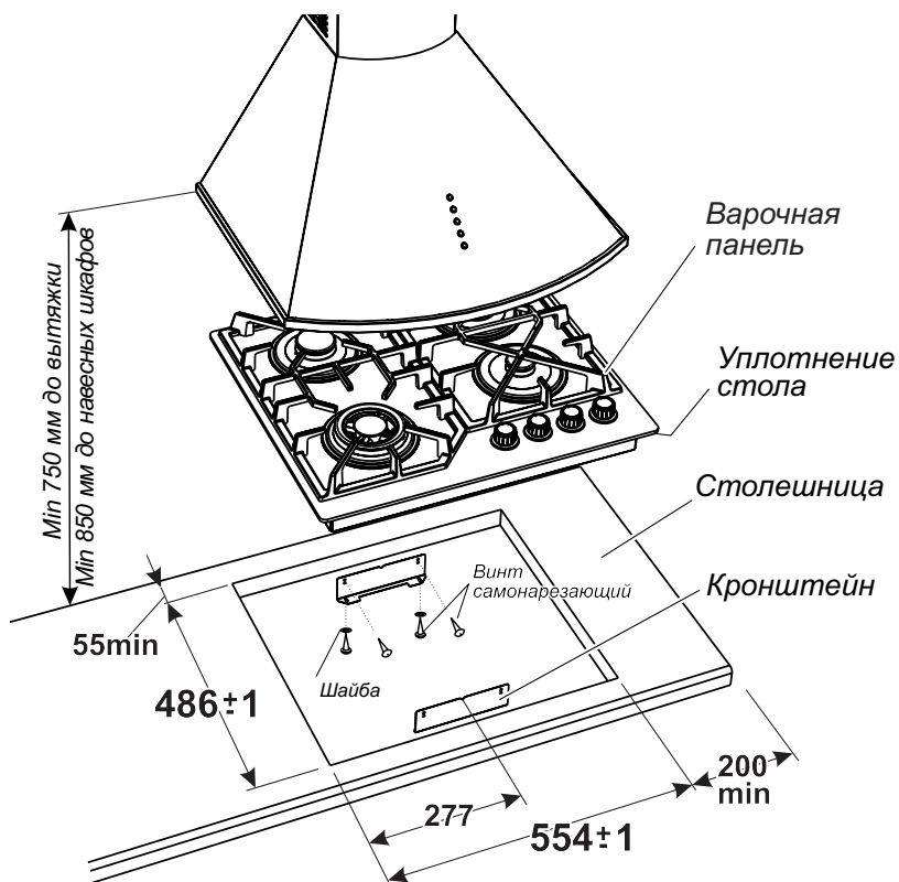
Рис. 12 МОДЕЛЬ ПВГ 2232, ПВГ 2232-01
