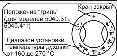
Ручка духовки плит моделей 5040.31г, 5040.33г, 5040.41г, 5040.43г
